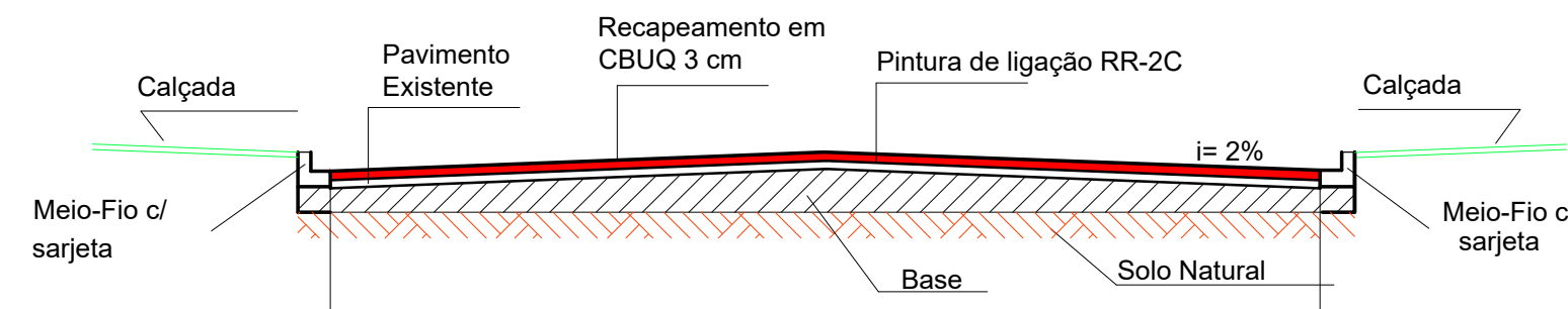
SEÇÃO TRANSVERSAL - RECAPEAMENTO SEM ESCALA
