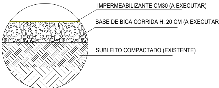
DETALHE RECONSTRUÇÃO DE BASE 3/ ESCALA
